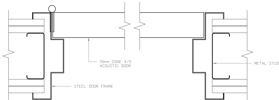
1 ZONE 4/5 DOOR/FRAME PLAN VIEW
